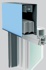
RAFF S Putz (Blendenhöhe 170 mm - 300 mm)
